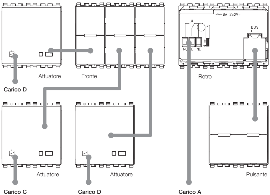
Apparecchio di comando a tre pulsanti semplici e attuatore (Eikon 20545; Arké 19545; Idea 16985; Plana 14545).
