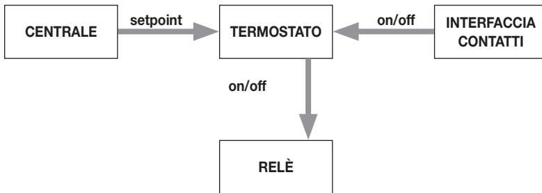
Figura 5.2.1.1: termostato con interfaccia contatti per forzatura in OFF del controllo clima
